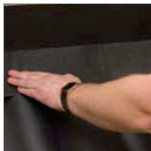
Inddækningsbåndet trykkes fast mod toppen af tagmaterialet.
