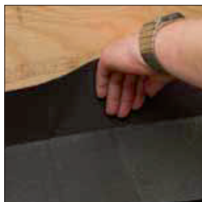
Inddækningsbåndet glattes og presses, så der kommer fuld vedhæftning.
